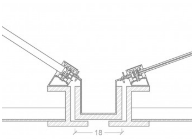
Dettaglio tecnico del sistema di fissaggio dei moduli, fornito da Ing. Klaus Fleischmann e ridisegnato da Eurac Research
